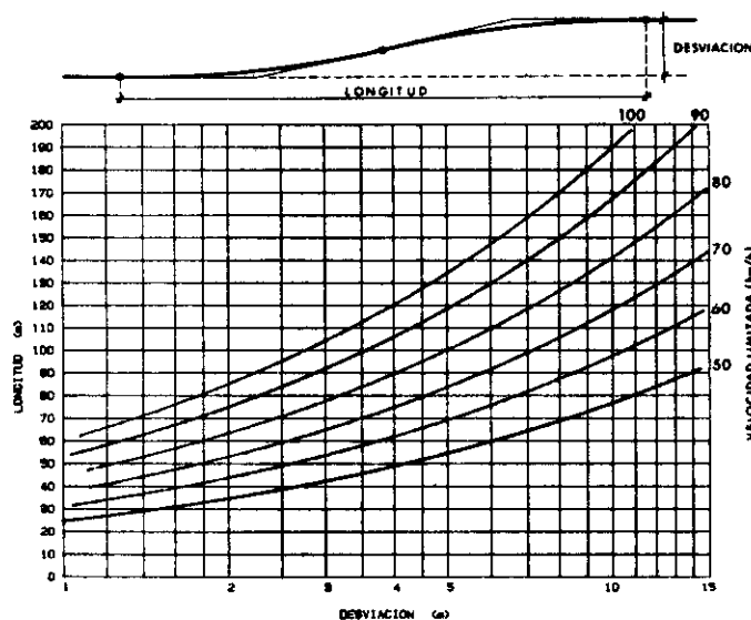
Fig. 34.—LONGITUD MÍNIMA PARA DESVÍO PARALELO DE UN CARRIL
