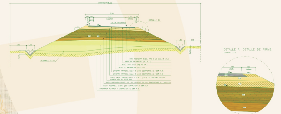
SECCIÓN TIPO RAMAL UNIDIRECCIONAL
